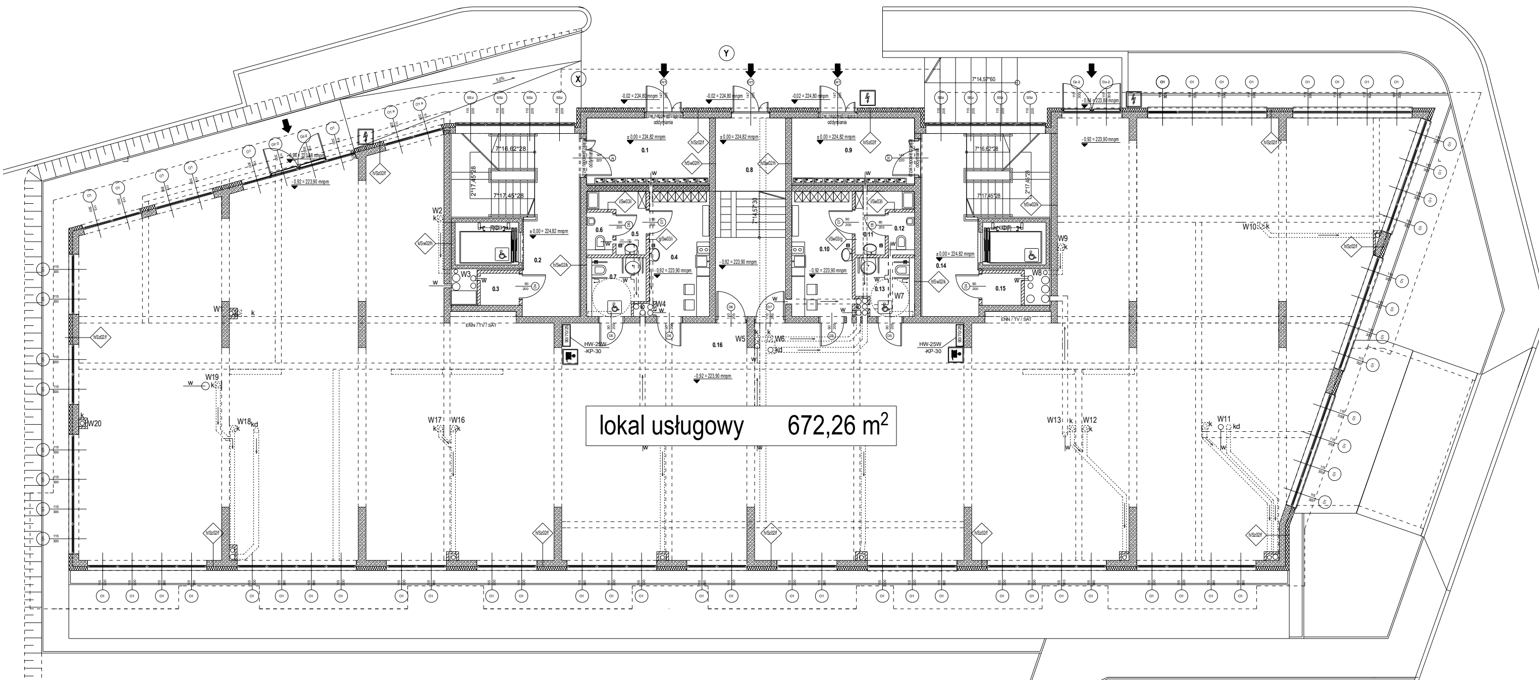
Rzut parteru
